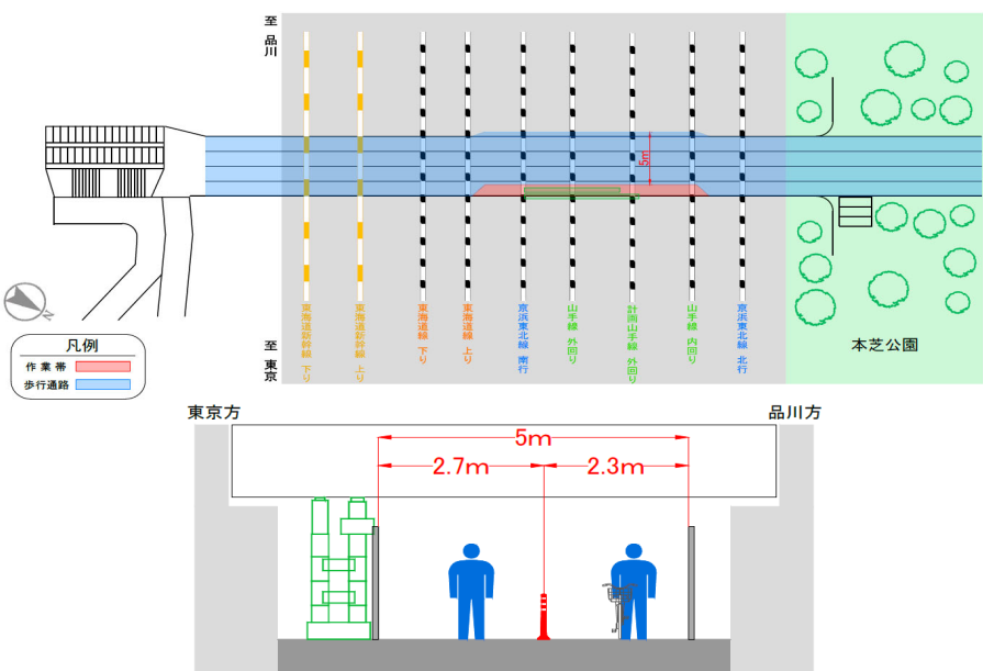
4-1 ベント設置両側施工時 規制図(6:00~22:00) 3月下旬~4月下旬
