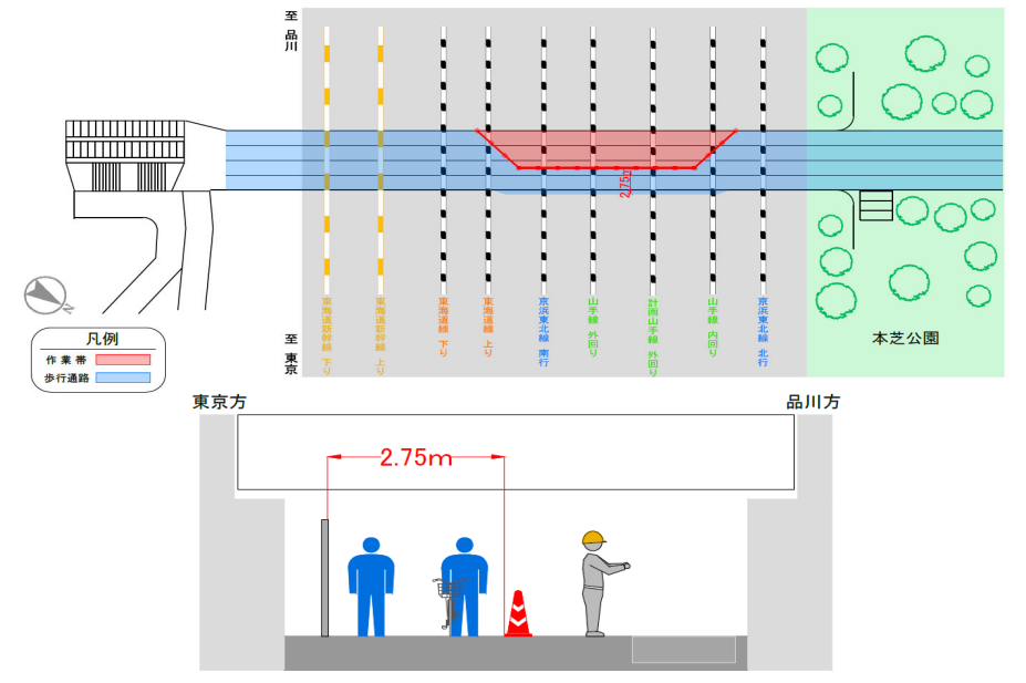
3-2 ベント設置施工時 規制図(22:00~6:00) 1月下旬~3月下旬
