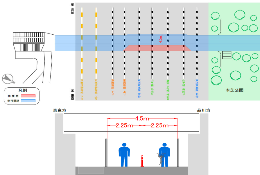
2-1 基礎コン品川方施工時 規制図(6:00~22:00) 1月中旬~1月下旬
