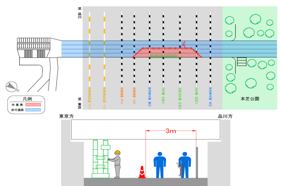
4-2 ベント設置両側施工時 規制図(22:00~6:00) 3月下旬~4月下旬
