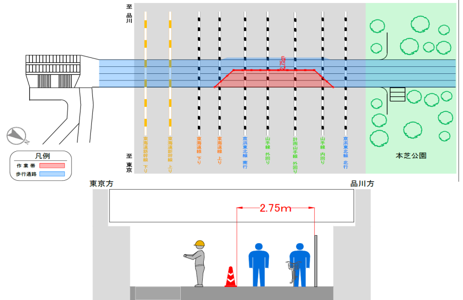
2-2 基礎コン品川方施工時 規制図(22:00~6:00) 1月中旬~1月下旬
