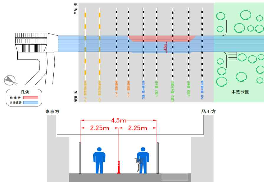
3-1 ベント設置施工時 規制図(6:00~22:00) 1月下旬~3月下旬
